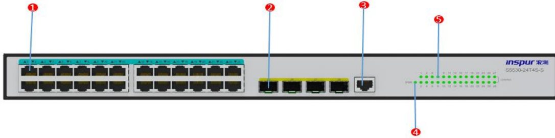
图 1-2 S5530-24T4S-S 前面板示意图
